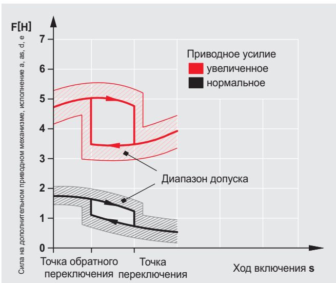
Диаграмма „сила-путь“ при переключении рычага с роликом. Исполнение S826 a, S826 as, S826 d, S826 e
