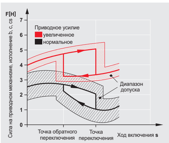
Диаграмма „сила-путь“ при переключении толкателя. Исполнение S826 b, S826 c, S826 cs
